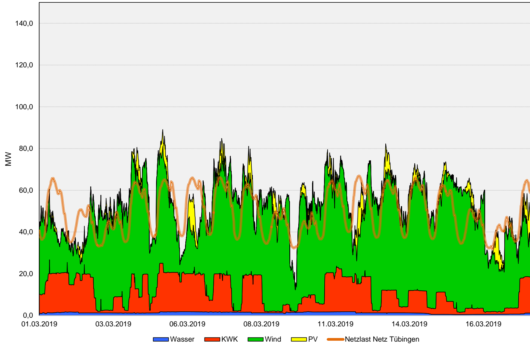
Netzlast im Vergleich zur Erzeugung 1.3.-18.3.19
