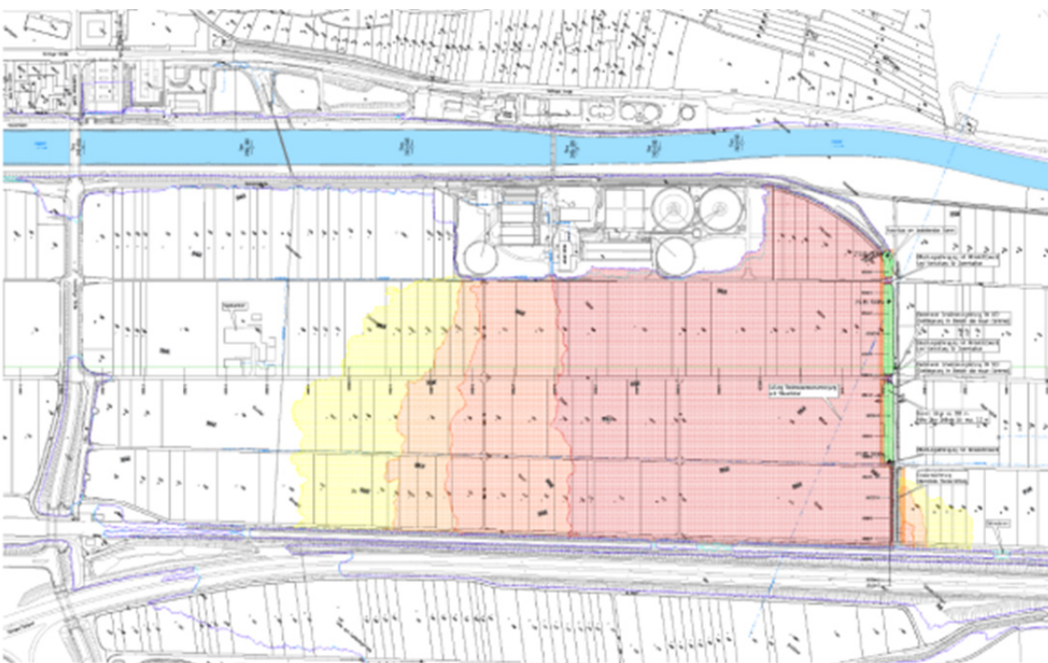
Lageplan der Maßnahme und der höher eingestauten Flächen (gelb-rot)
