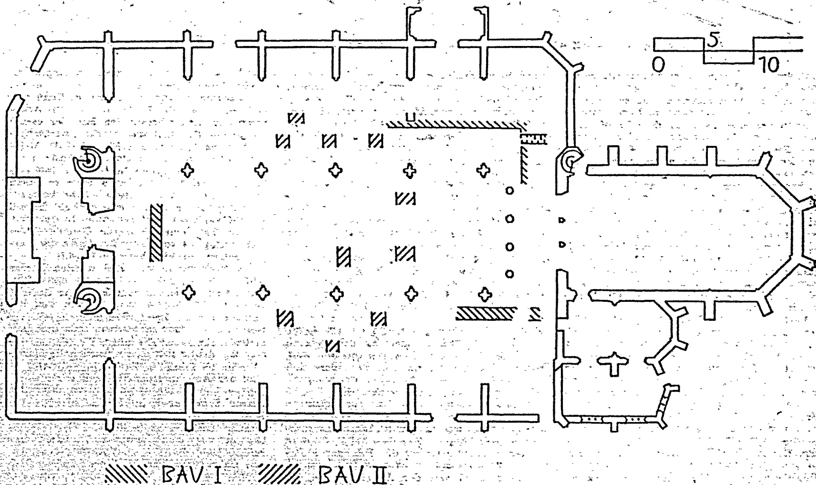
Abb. 1. Situationsplan des 1962 aufgedeckten Mauerwerks innerhalb der spätgotischen Hallenkirche nach dem Aufmaß von Arch. A. Achstetter.
