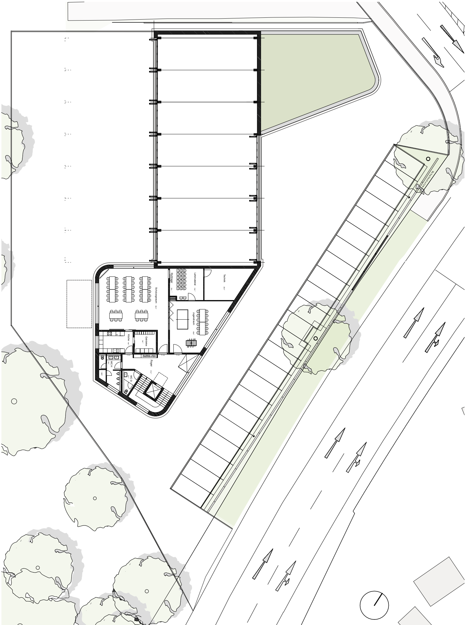
Neubau Feuerwehrhaus Lustnau, Entwurf Grundriss OG
