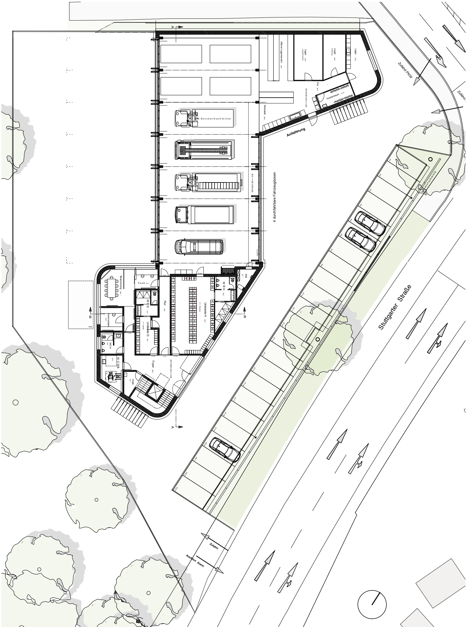
Neubau Feuerwehrhaus Lustnau, Entwurf Grundriss EG
