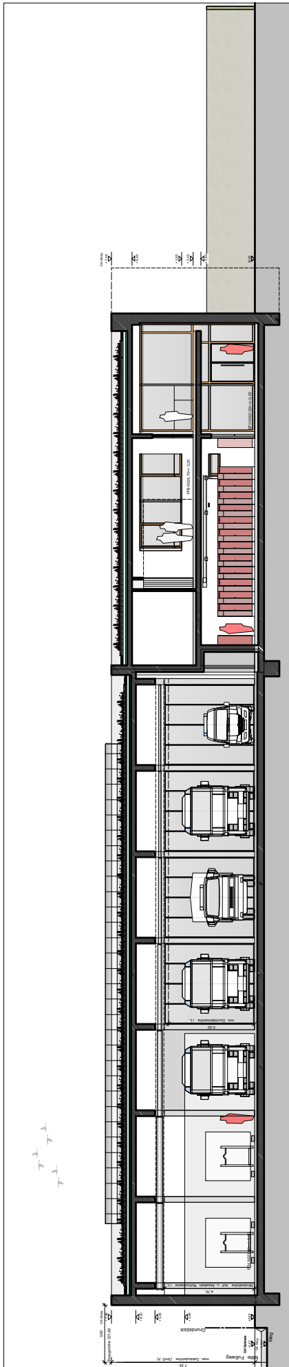
Schnitt A-A
