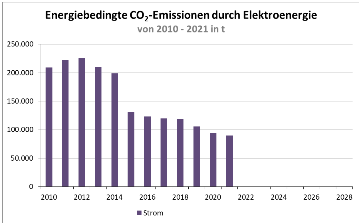
Abbildung 3: Absolute energiebedingte CO 2 -Emissionen (inkl. Vorketten) von 2010 - 2021 in t für den Energiesektor Strom
