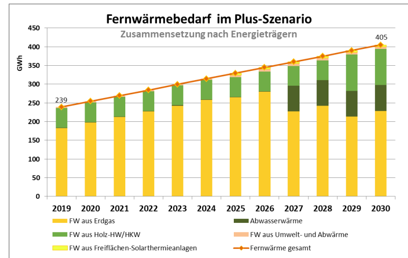
Abbildung 25: Prognose Fernwärmeverbrauch im Plus-Szenario
