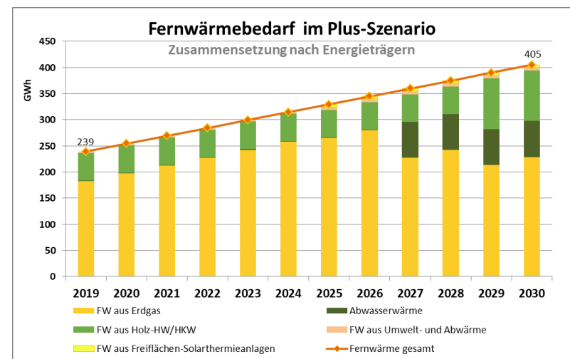
Abbildung 25: Prognose Fernwärmeverbrauch im Plus-Szenario
