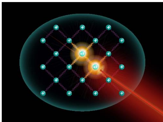
Illustration Ionenkristall: Andreas Müller
